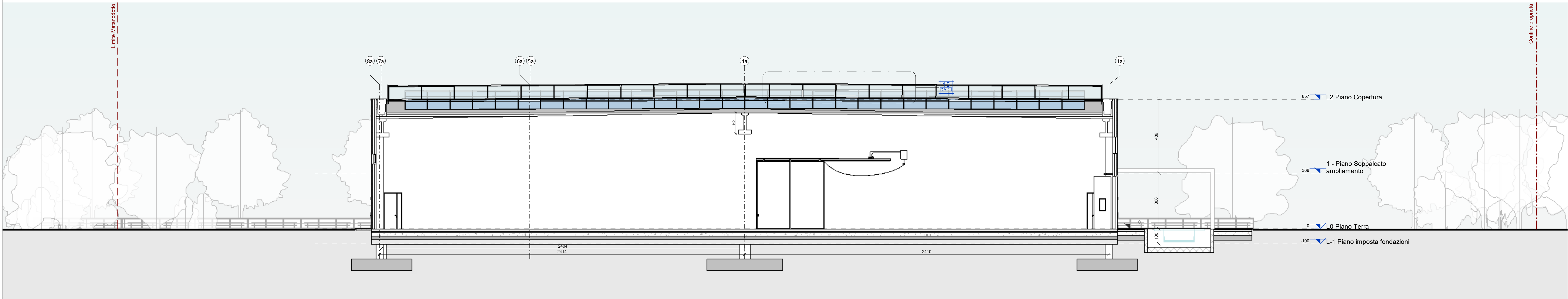
Sezione AA 1 : 100
