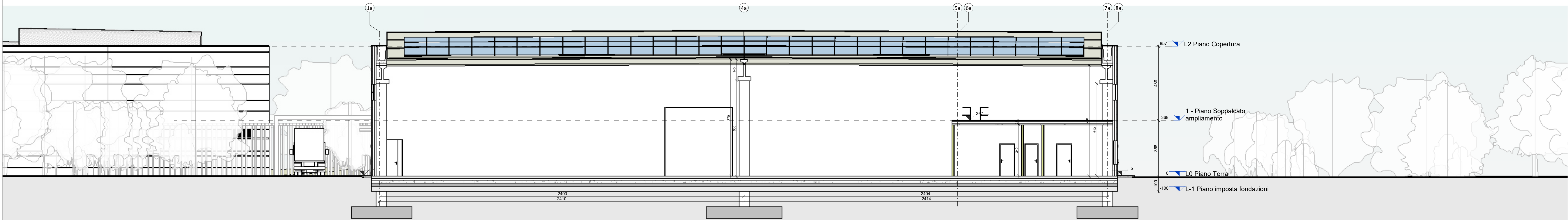
Sezione BB 1 : 100
