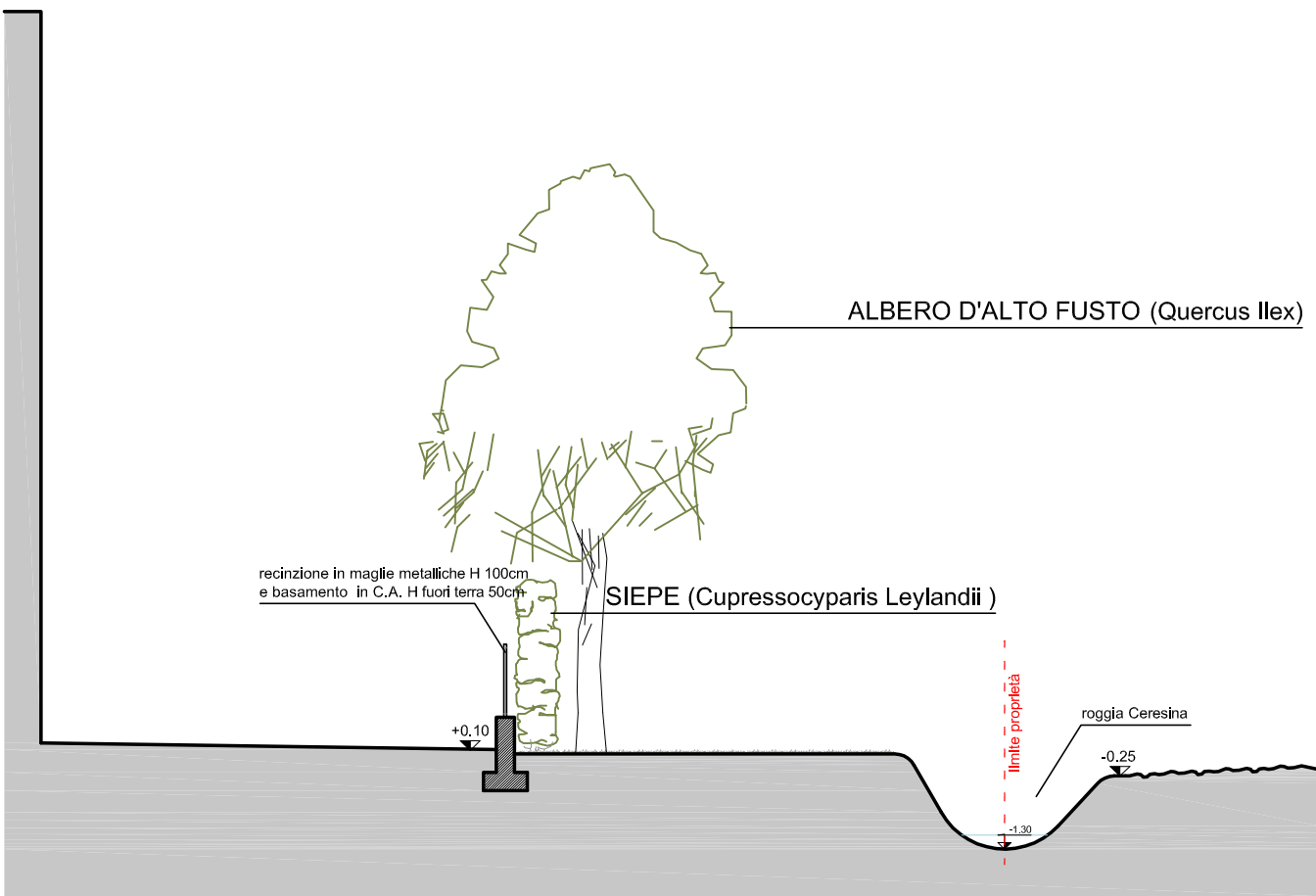
SEZIONE AA
