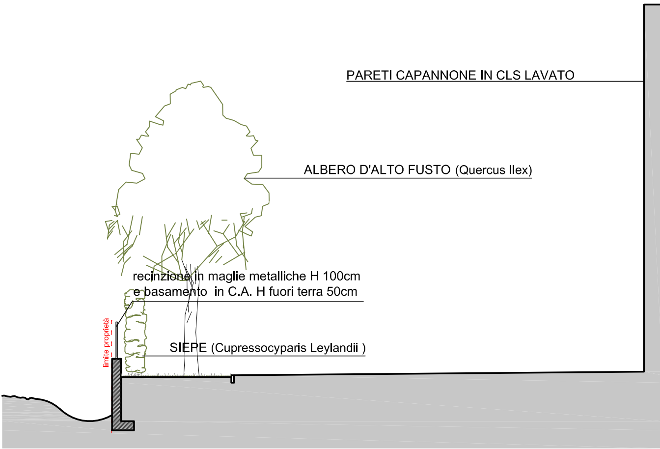
SEZIONE CC
